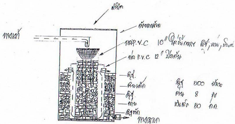
แบบประยุกต์
