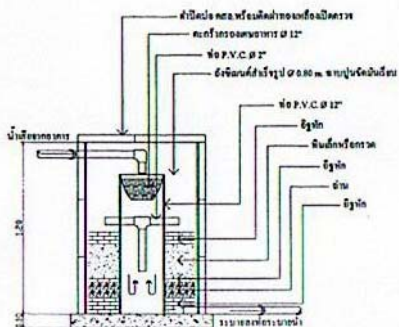
แบบบ่อคักใจมัน กรณีเป็นดัชชีมันค้ำเจ้ารูป
