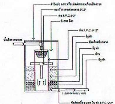
แบบบ่อนักใจมั่น กรณีเป็นถึง 200 ถึง
